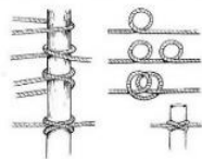
巻き結び (クラブヒッチ)
